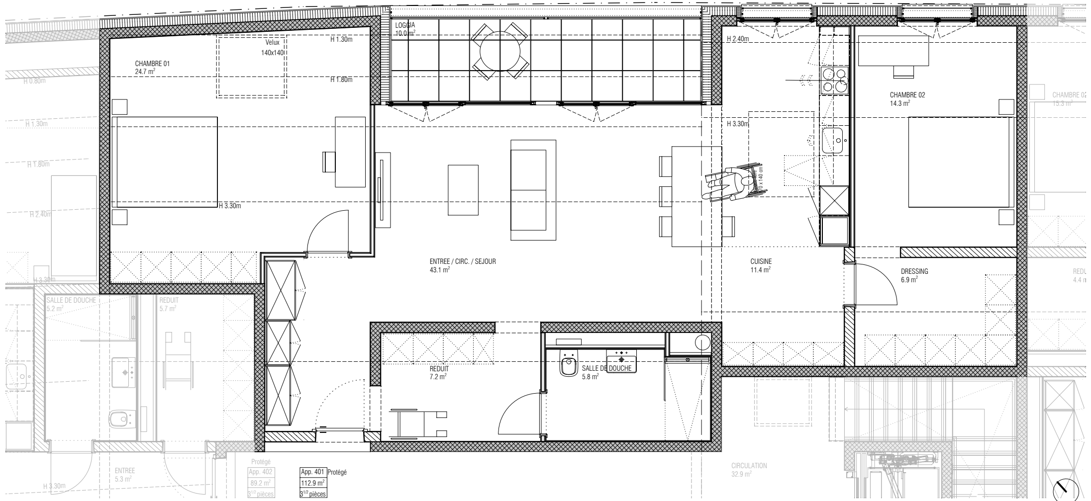
APPARTEMENT PROTEGE N° 401 - NIVEAU 04
