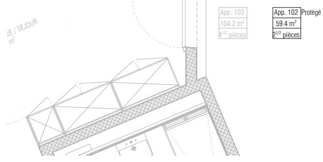
APPARTEMENT PROTEGE N° 102 - NIVEAU 01
